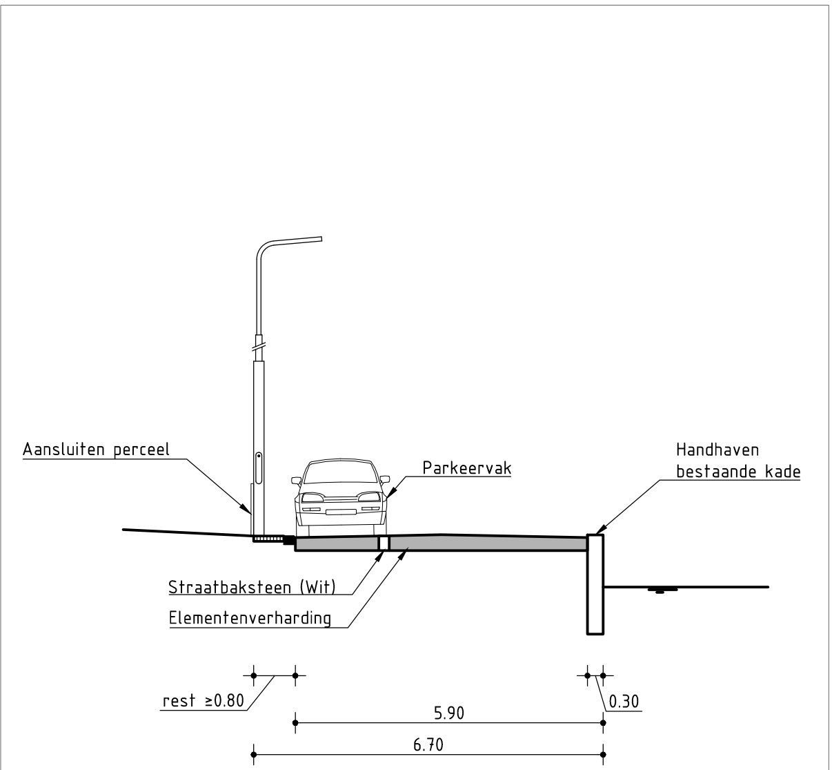
PRINCIPE DWARSPROFIEL A Parkeren + tweerichtingsverkeer auto/Fiets Schaal 1:100
