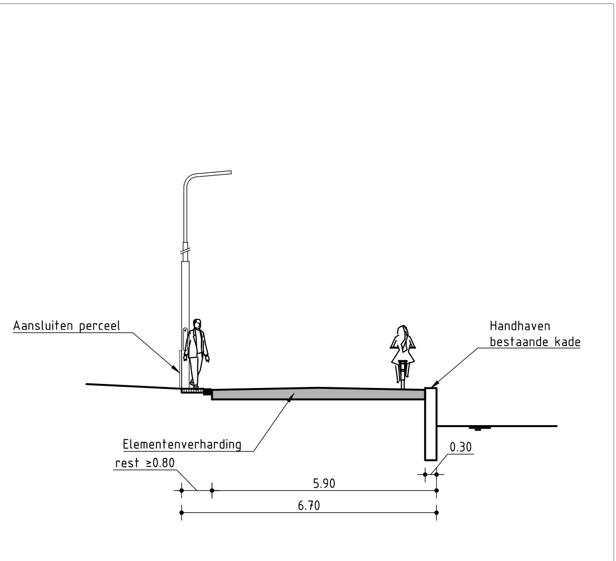
PRINCIPE DWARSPROFIEL B Zonder parkeren + tweerichtingsverkeer auto/Fiets (passeertociale) Schaal 1:100
